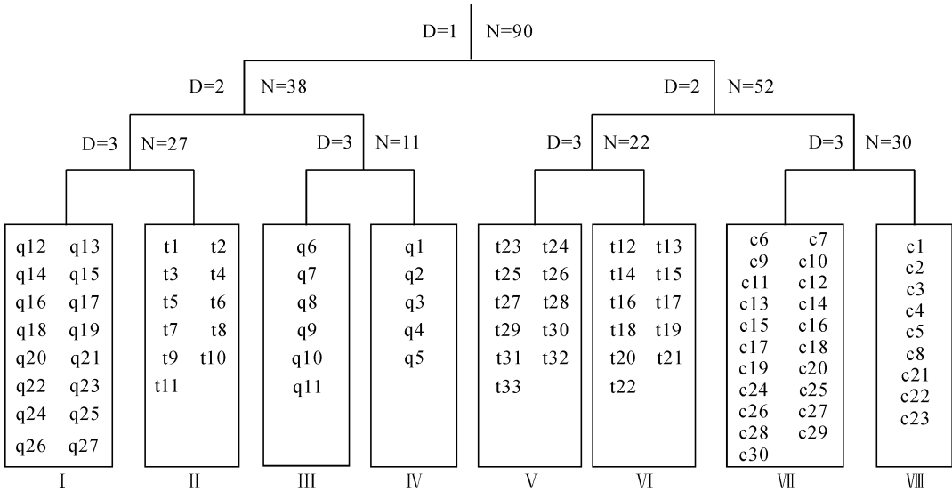
图 1 TWINSpan 分类结果树状图
