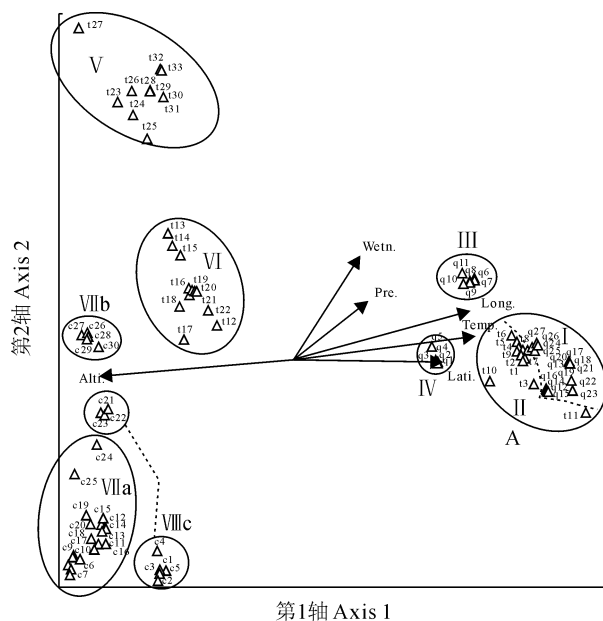
图 2 紫花针茅草原 90 条样带及环境因子的 CCA 排序图
